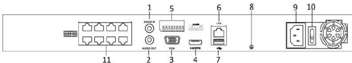
背面図
