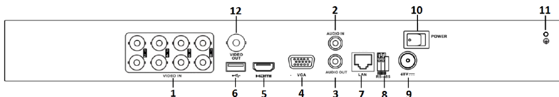
背面図
